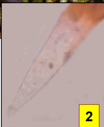
1 : Spores 5-6 x 4-5 \mu\text{m} , elliptiques, à apicule de grande taille. 2 : Cheilocystides et pleurocystides, 50-100 x 10-25 \mu\text{m} , largement fusoides et atténuées en pointe.
